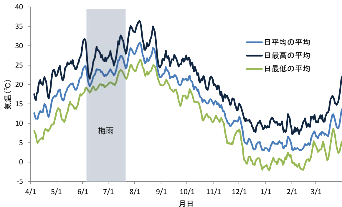
図 6 平成 26 年度全調査地点の日平均気温、日最高気温、日最低気温の平均値の推移 (5 日移動平均)
