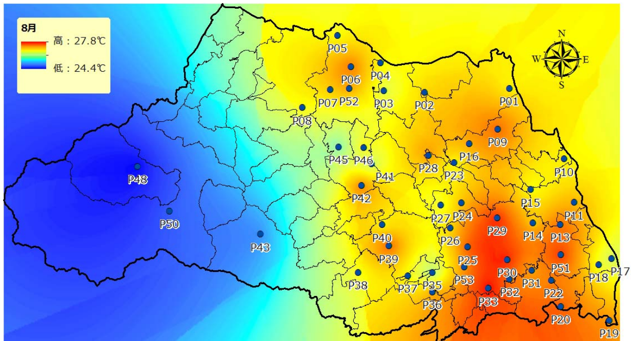
图 12 气温分布（平成 26 年 8 月平均）
