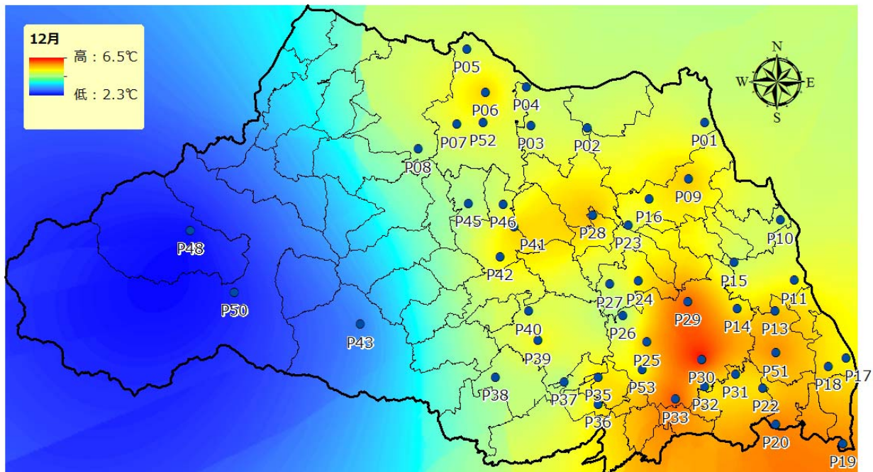
図 16 気温分布（平成 26 年 12 月平均）
