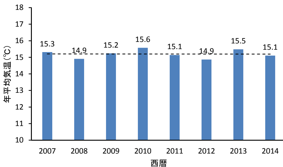
図 21 全調査地点年平均気温の推移
