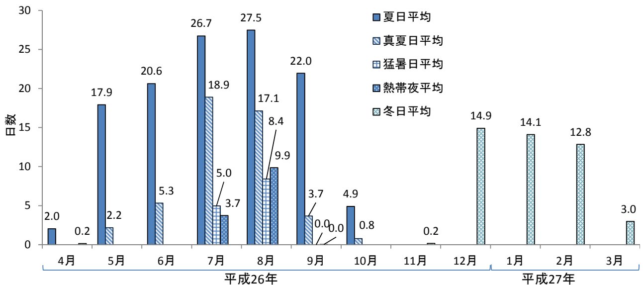
図 7 平成 26 年度の夏日、真夏日、猛暑日、熱帯夜、冬日日数の全調査地点月別平均値
