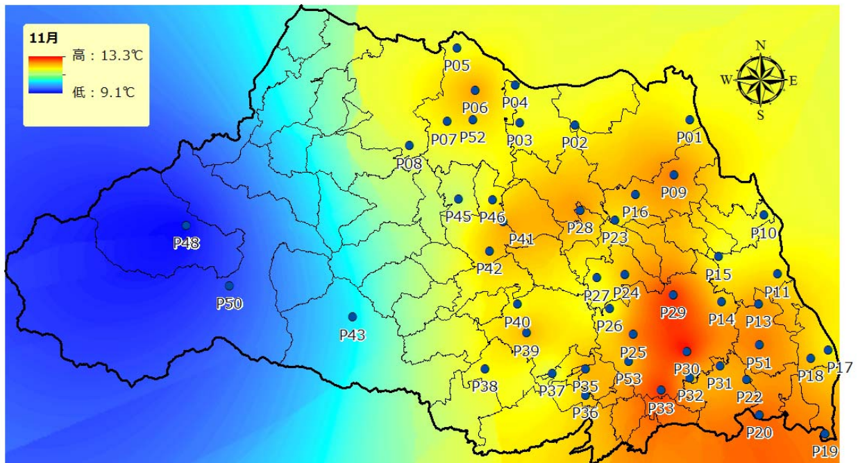
図 15 気温分布（平成26年11月平均）
