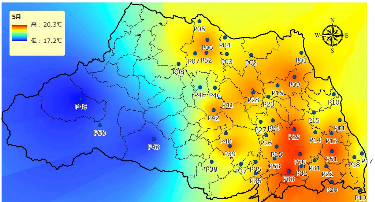
図 9 気温分布（平成 26 年 5 月平均）
