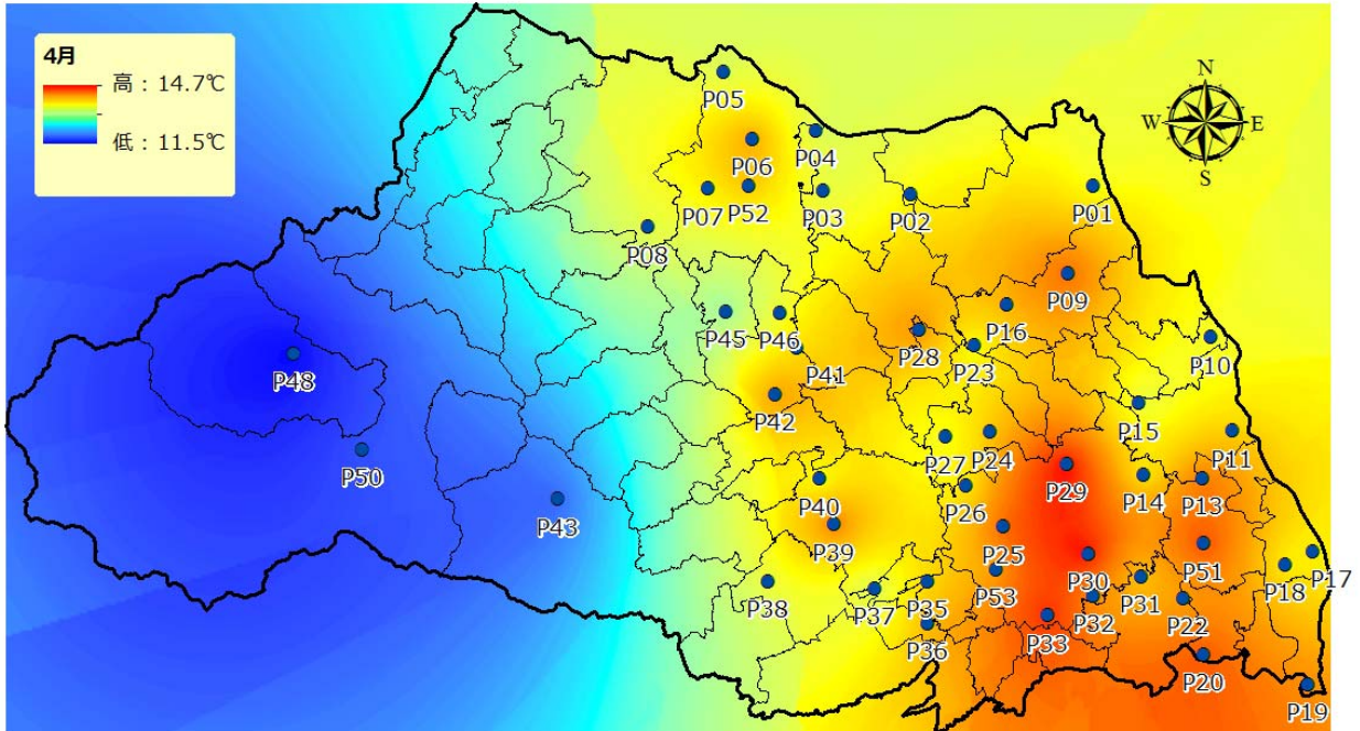
図 8 気温分布（平成 26 年 4 月平均）
