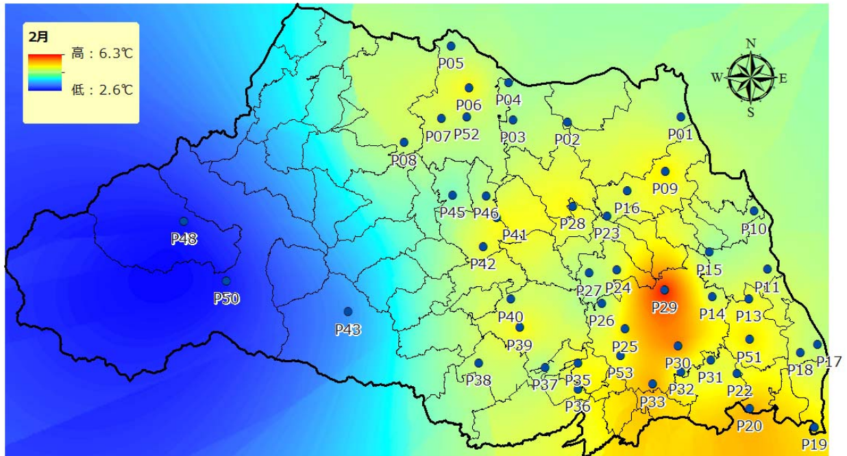
图 18 气温分布（平成 27 年 2 月平均）
