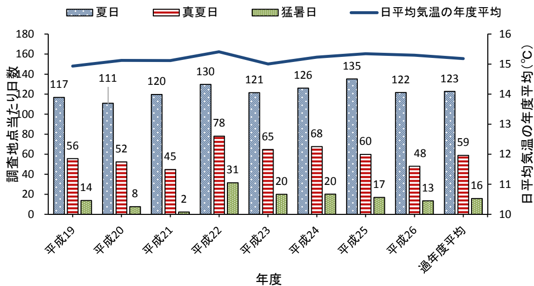
図 24 年度別、夏日、真夏日、猛暑日日数の全調査地点平均値の推移
