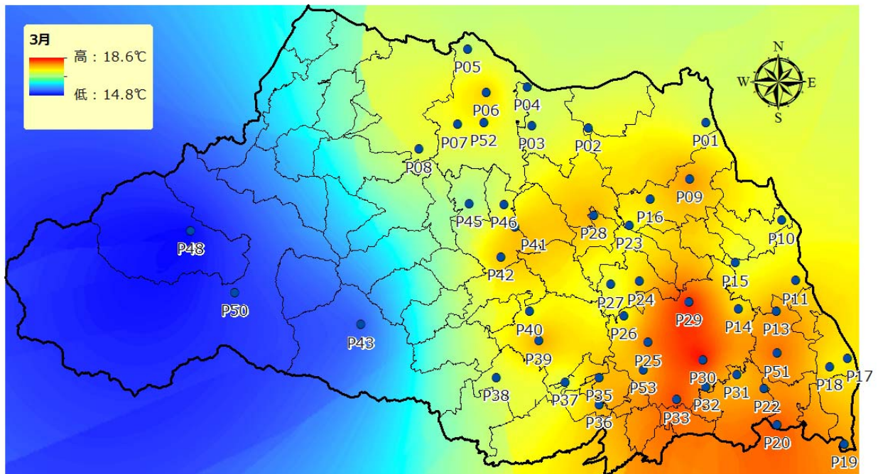
图 19 气温分布（平成 27 年 3 月平均）
