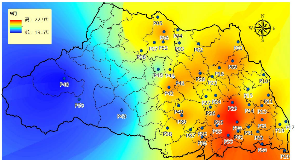
图 13 气温分布（平成 26 年 9 月平均）
