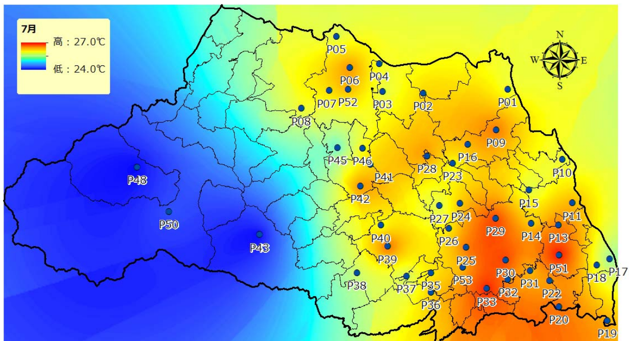
图 11 气温分布（平成 26 年 7 月平均）
