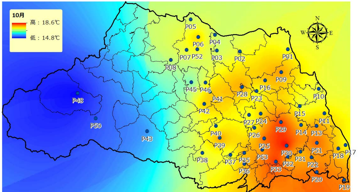
図 14 気温分布（平成26年10月平均）
