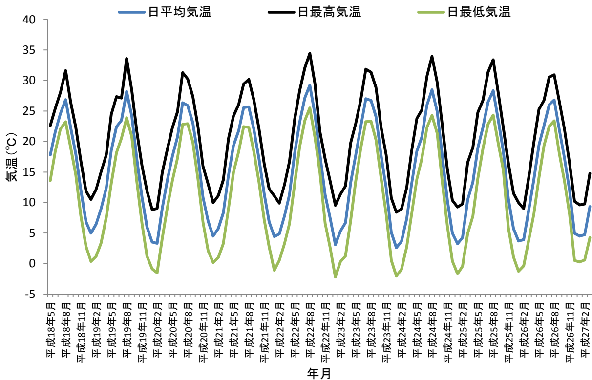
図 20 日平均気温、日最高气温、日最低气温の全調査地点月平均の推移
