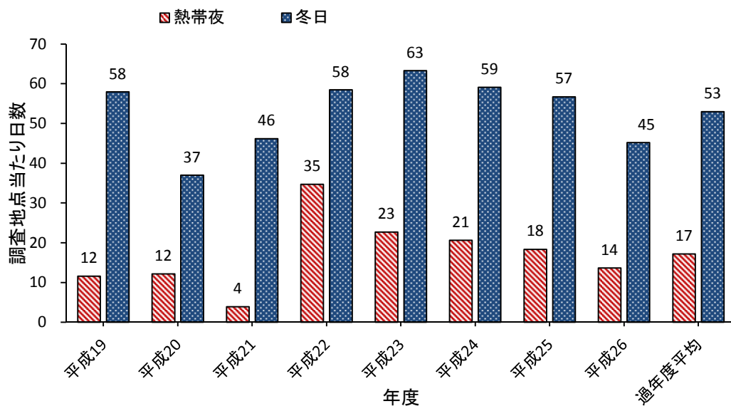
図 25 年度別、熱帯夜、冬日日数の全調査地点平均値の推移
