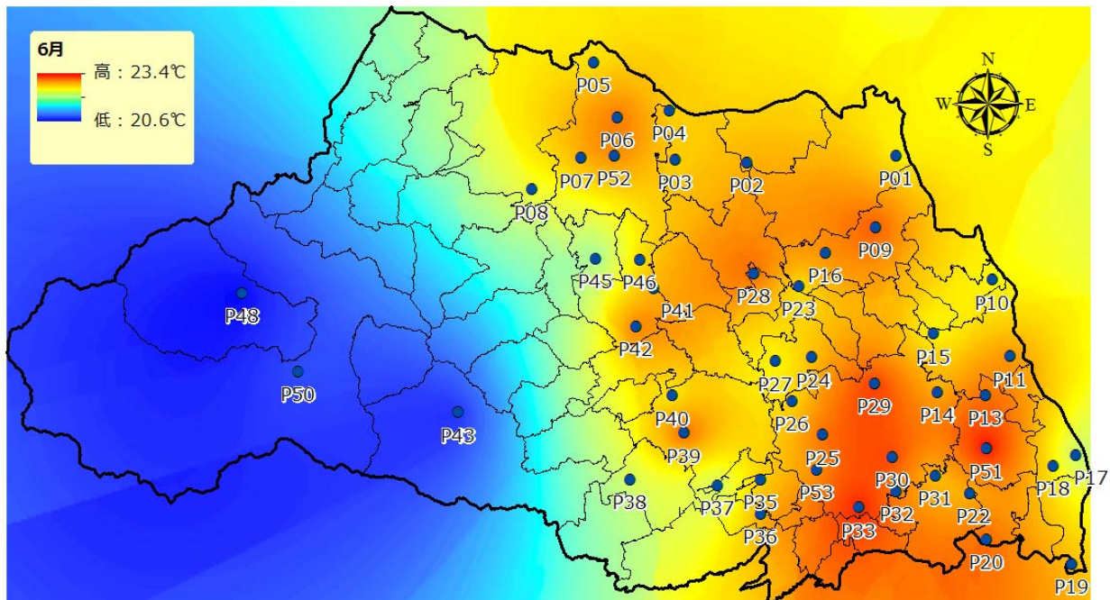
图 10 气温分布（平成 26 年 6 月平均）
