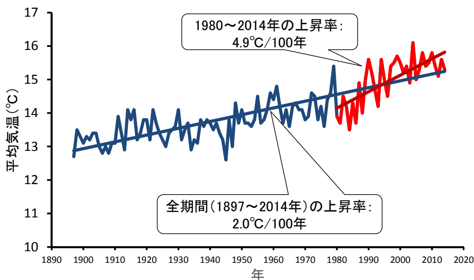
図 1 埼玉県の年平均気温の推移(熊谷気象台)
